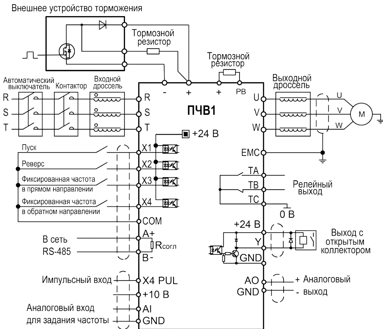
Рисунок 6.7 – Общая схема подключения ПЧВ мощностью 7,5 кВт и выше
