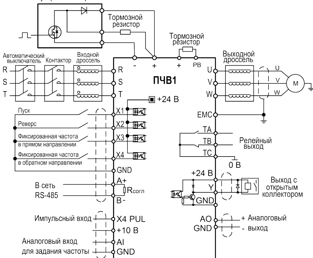
Рисунок 6.6 – Общая схема подключения ПЧВ мощностью до 7,5 кВт
