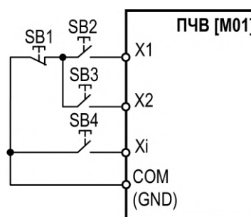
Рисунок 6.10 – Трехпроводная схема управления 1 (F05.20 = 2)
